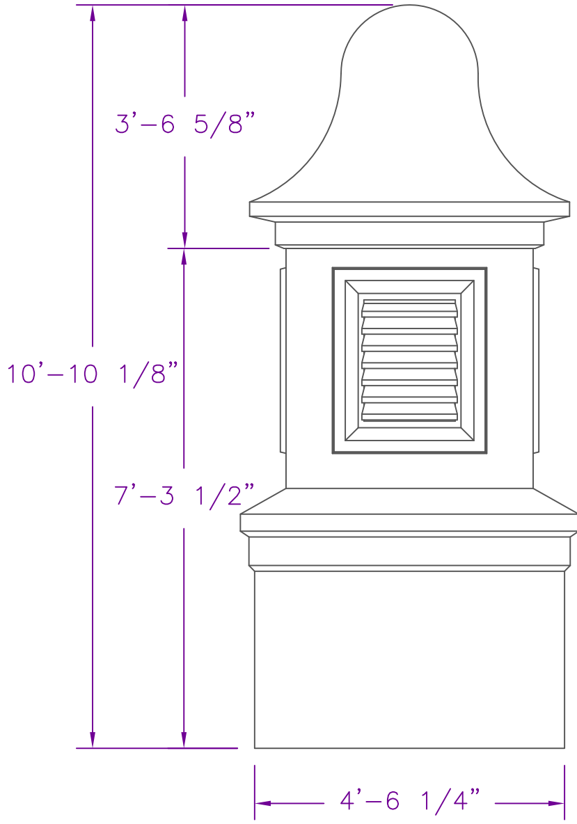
1 ELEVATION E1
