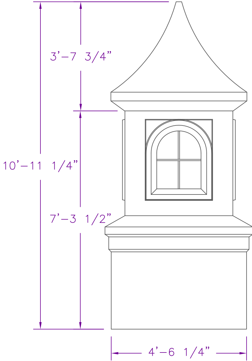
1 E1 ELEVATION
