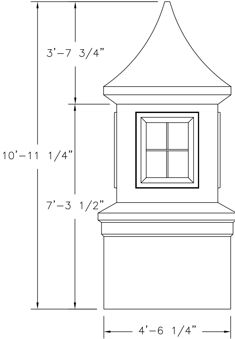
1 E1 ELEVATION
