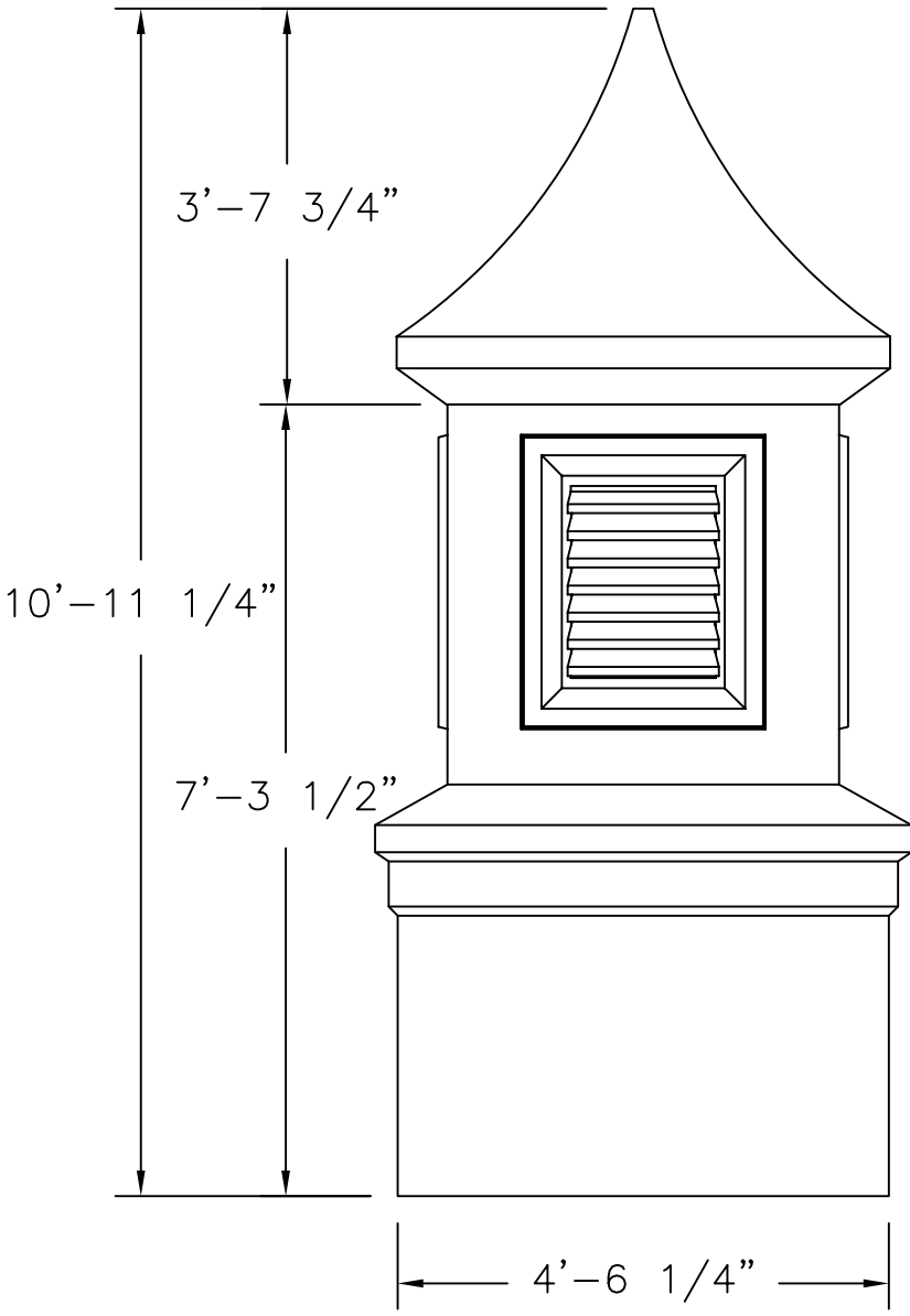
1 E1 ELEVATION
