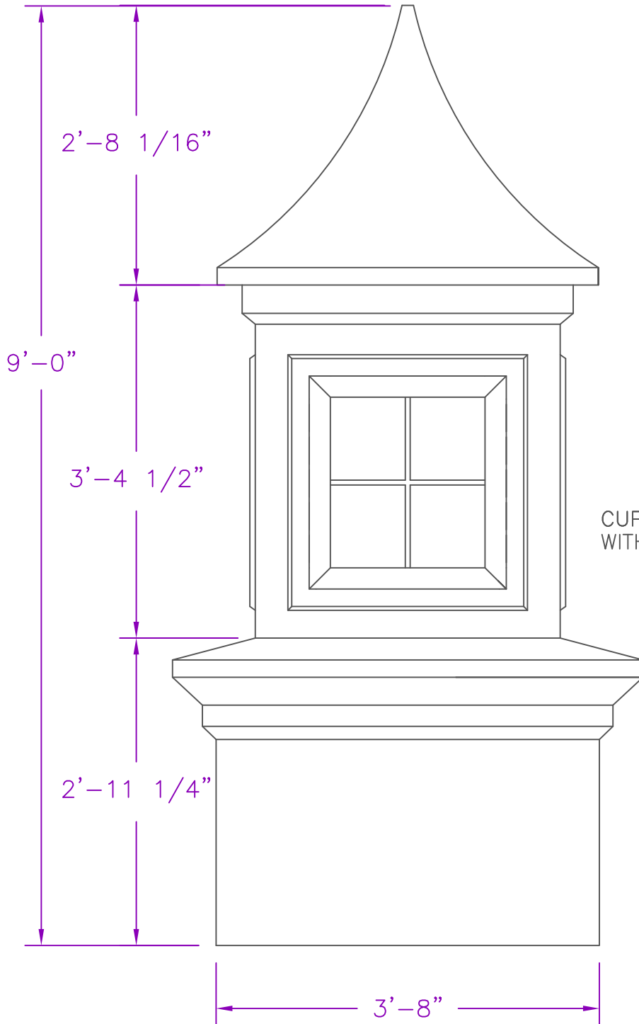
1 E1 ELEVATION
