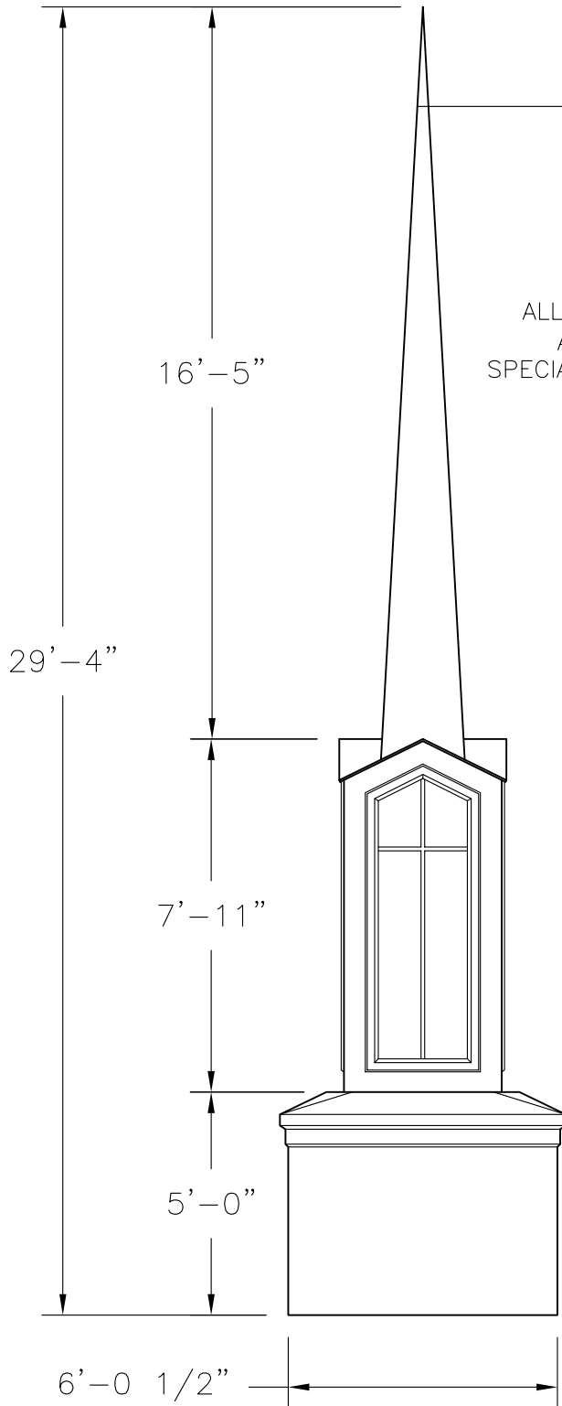
① ELEVATION E1
